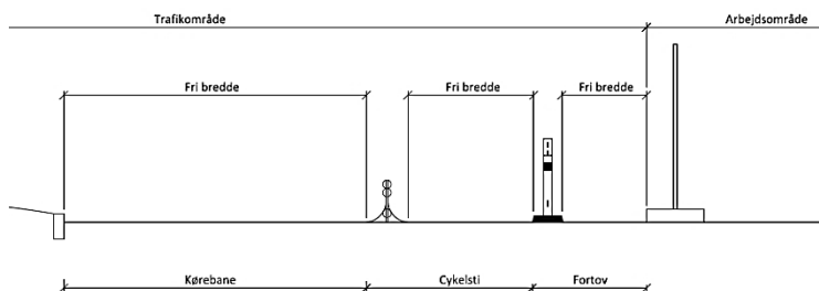
Figur 2.10 Måleregel for fri bredde.
