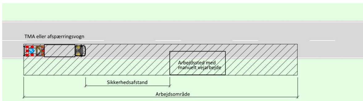
Figur 7.37 Princip for sikkerhedsafstand for vejarbejdere mellem TMA/afspærringsvogn og arbejdssted.
