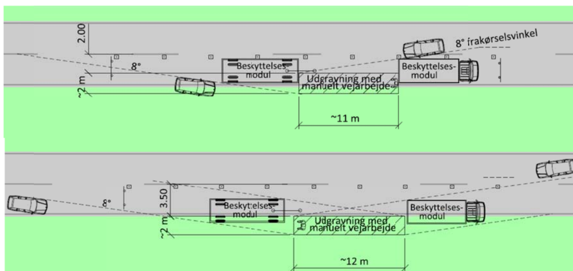
Figur 3.5 Eksempler på anvendelse af beskyttelsesmodul (beskyttelsesniveau 4) ved udgravning med manuelt vejarbejde i eller tæt på kørebanen på en 2-sporet vej. Beskyttelsesmodulernes placering tilpasses udgravningens længde og bredde. Færdselsregulering er ikke vist fuldt ud.
