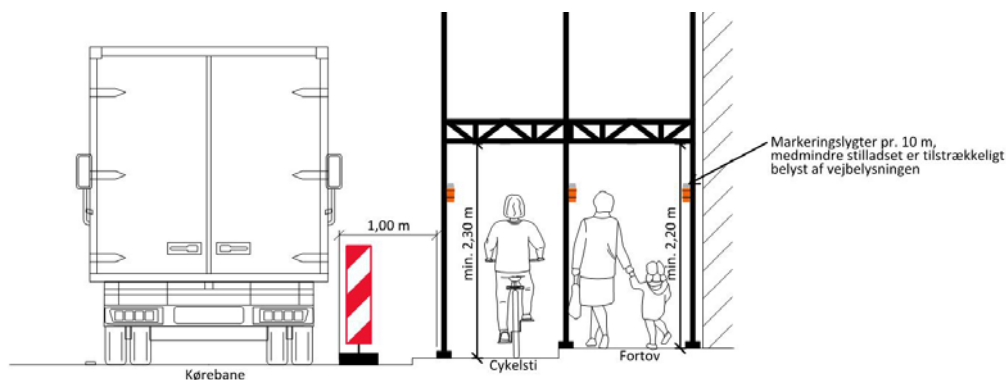
Figur 6.1 Eksempel på afmærkning af stillads på cykelsti og fortov med stilladsben under 1 m fra kørebane.
