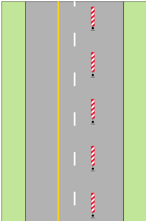
Figur 6.1. Eksempel hvor hvid kørebaneafmærkning ikke skal fjernes. (Principskitse der ikke er gældende for konkret afmærkning).
