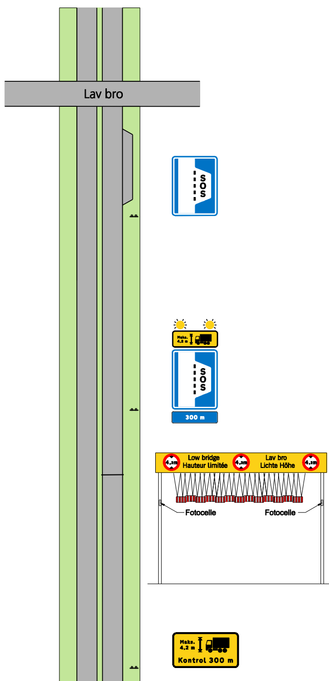
Figur 5.1. Placering af tavler i forbindelse med midlertidig højdebegrænsning af bro eller lignende.
