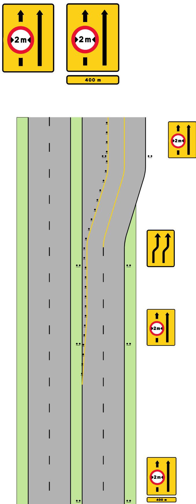
Figur 3.3. Eksempel på anvendelse af E 16 Vognbaneforløb.
