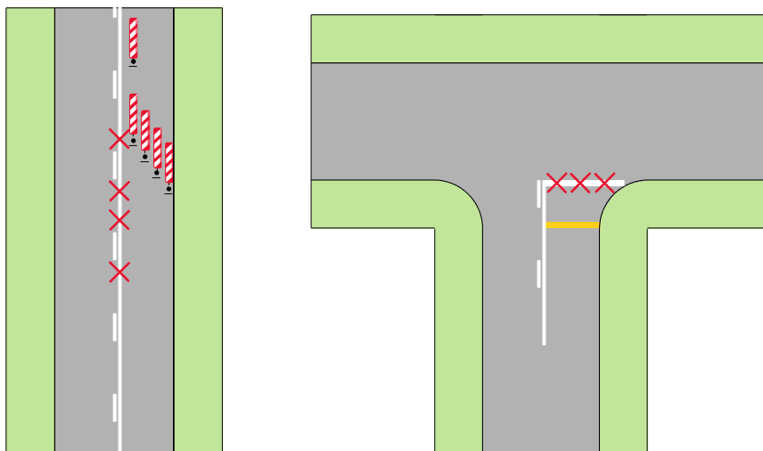
Figur 6.2. Eksempel hvor hvid kørebaneafmærkning skal fjernes eller tildækkes. (Principskitse der ikke er gældende for konkret afmærkning).
